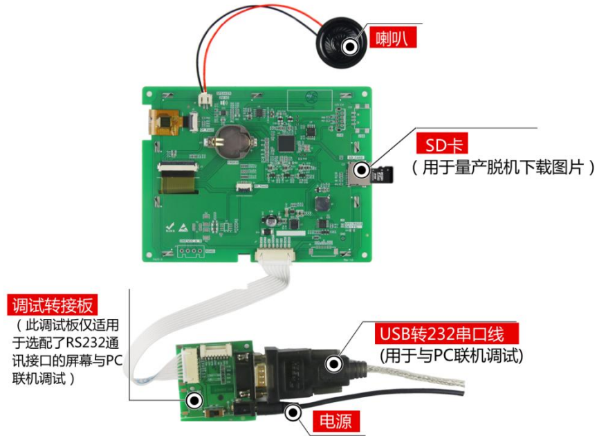
图 1-5 调试工具图
